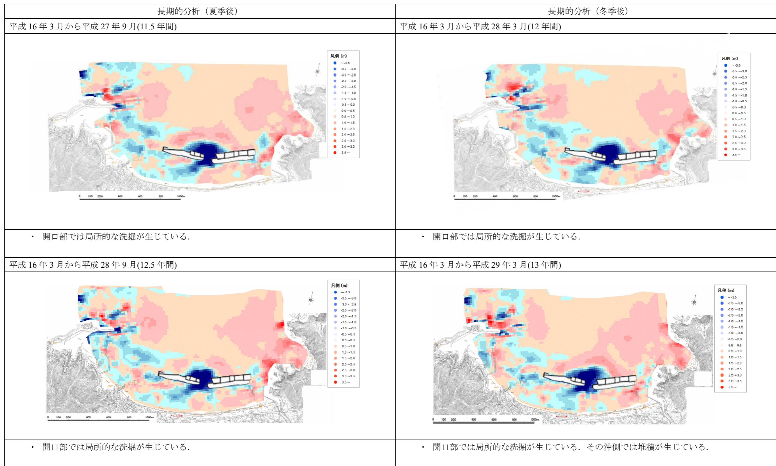
図 3.3.11 岩美海岸（浦富地区）の標高差分図(平成 16 年 3 月を基準とした長期的分析)
