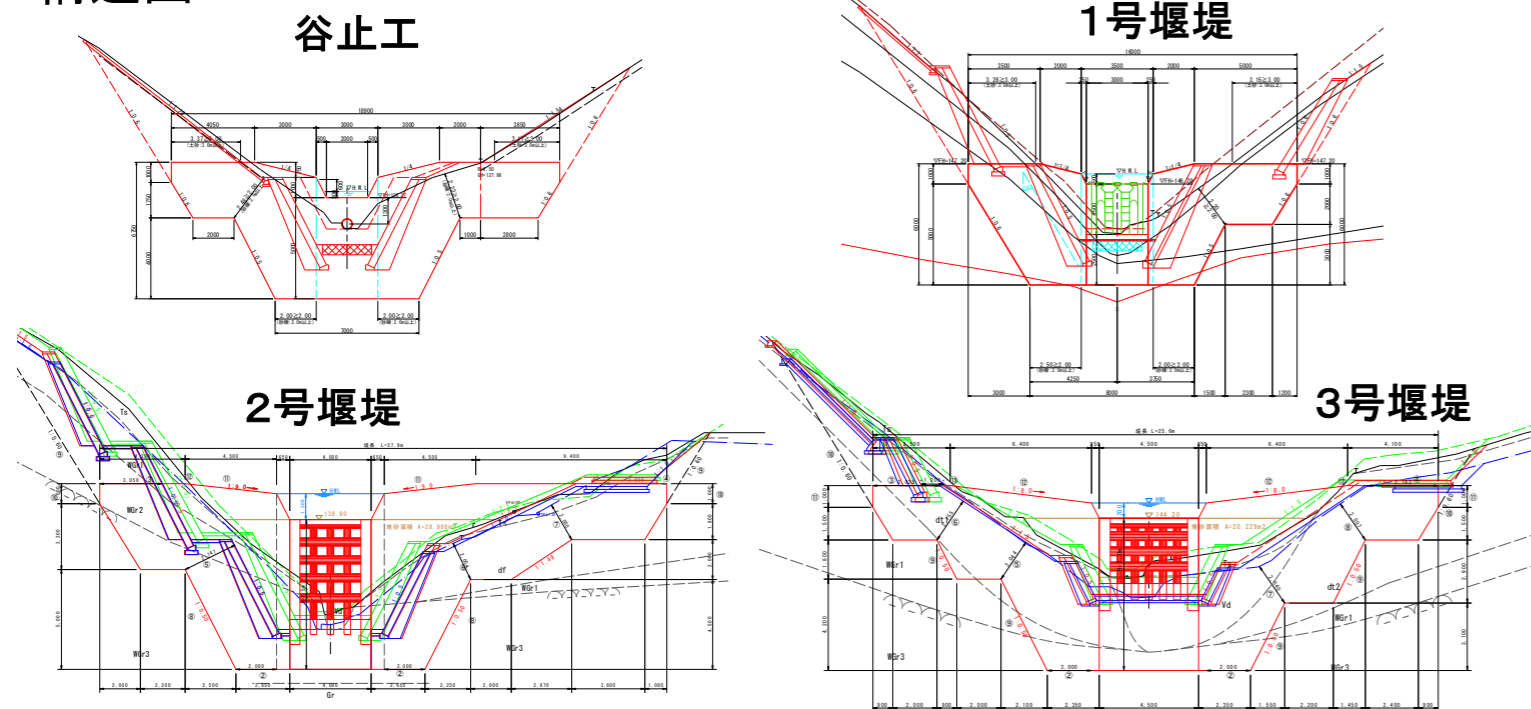
構造図
