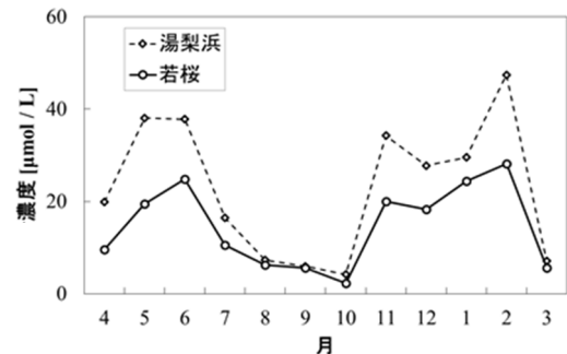
図6 降水中nss-SO 4 2- 濃度の経月変化
