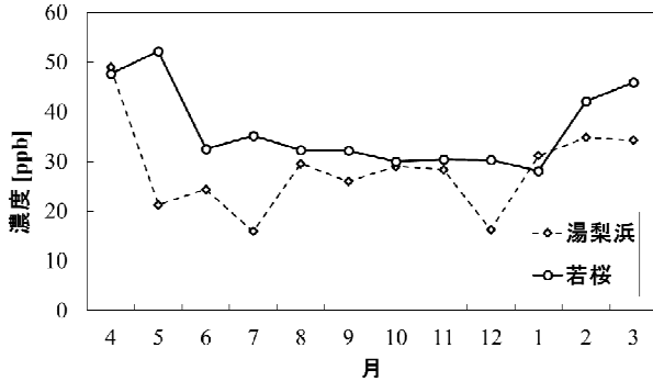
図 8 乾性沈着オゾン ( O_3 ) 濃度の経月変化
