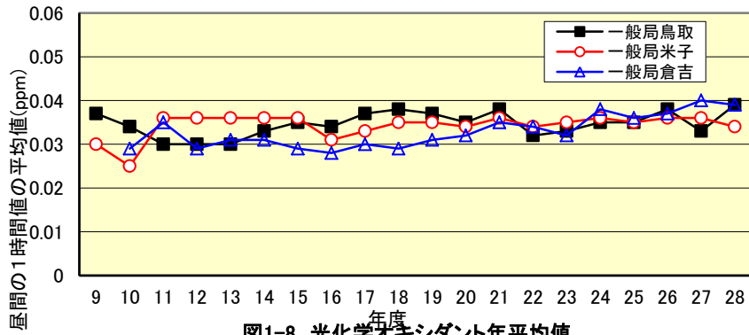
図1-8 光化学オキシダント年平均値
