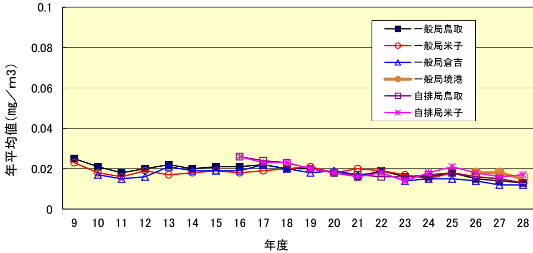
図1-3 浮遊粒子状物質の年平均値
