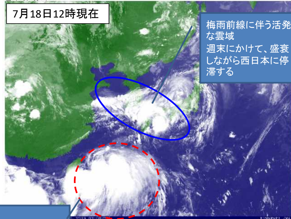
台風の雲の様子
