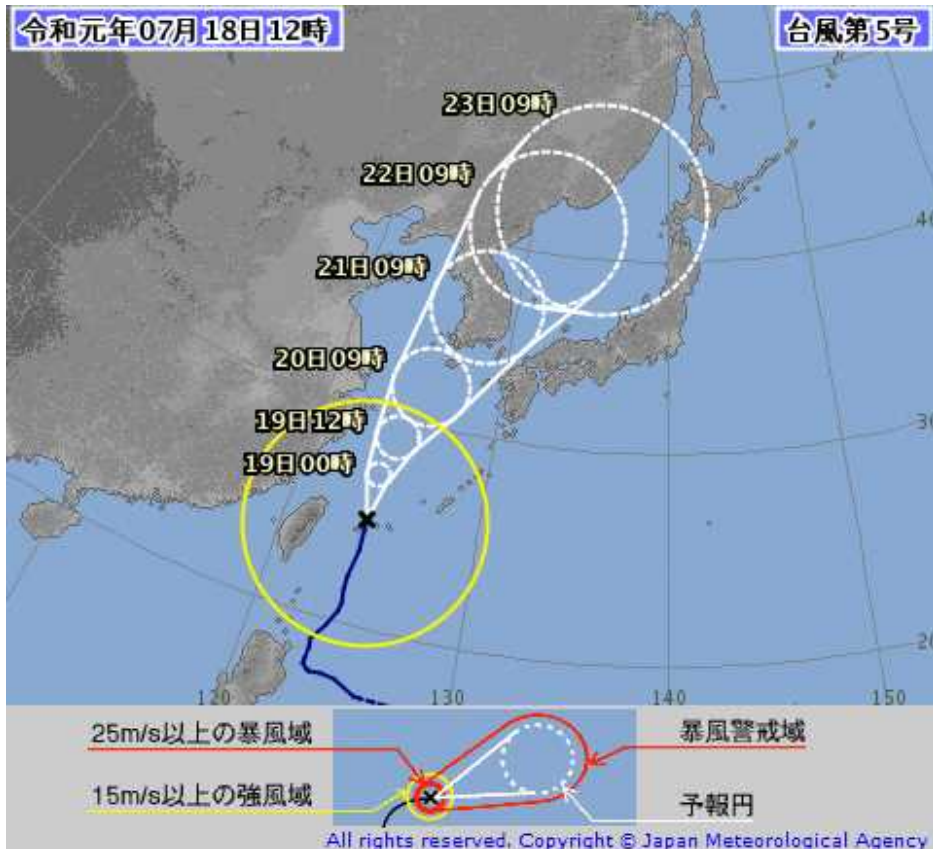
台風予想経路図
