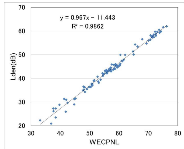
図4 Lden と WECPNL との相関(N=101)
