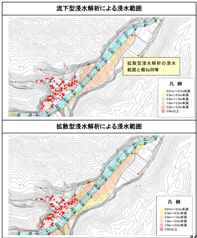
※1級水系 野坂川での浸水解析結果
