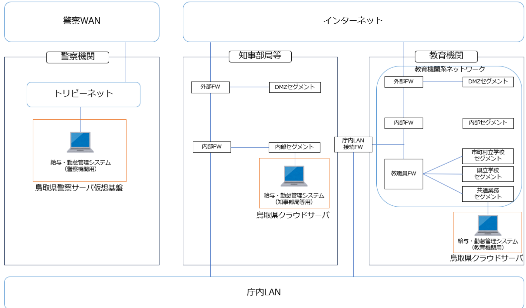
(参考 3) 現行のネットワーク概念図
