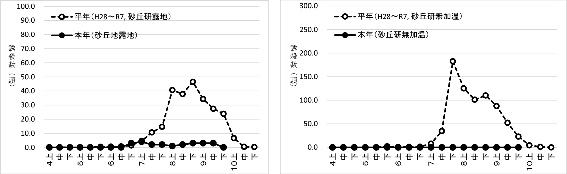
図2 黄色粘着板におけるチャノキイロアザミウマの誘殺消長
