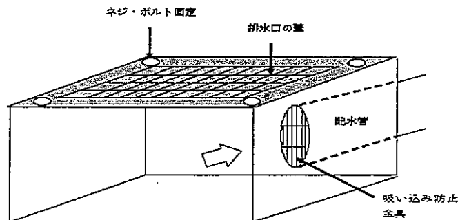
プールの排水口の例
