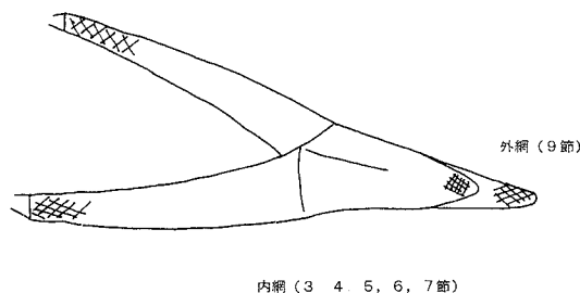
図1 網目選択試験漁具図
