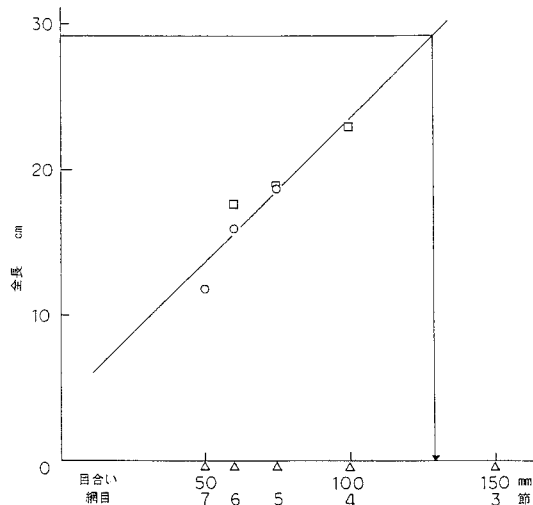
図4 各目合と50%網目選択率を示す体長との関係 (○:ソウハチ、□:ムシガレイ)
