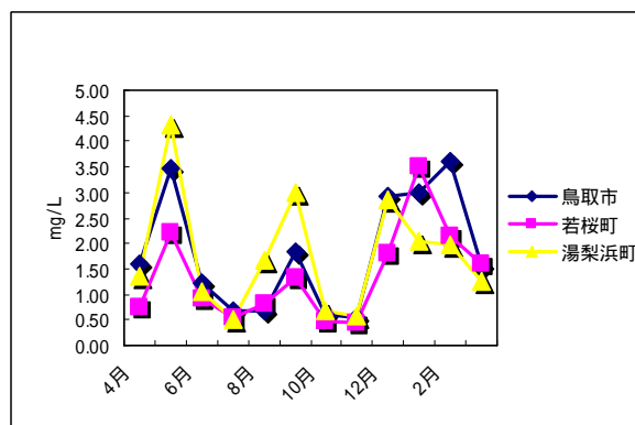
図3 平成21年度における NO 3 - 濃度の経月変化
