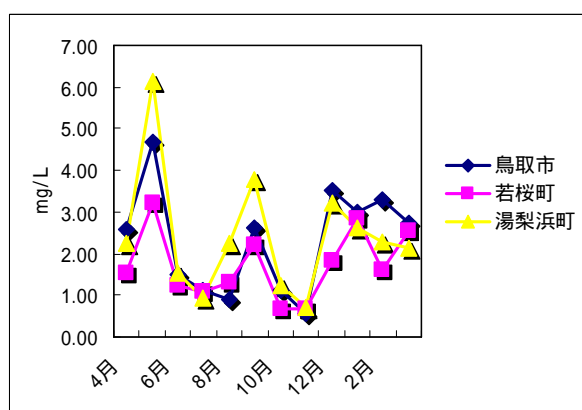
図2 平成21年度における nss-SO 4 2- 濃度の経月変化
