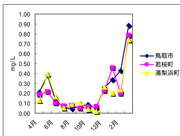
図4 平成21年度における nss-Ca 2+ 濃度の経月変化
