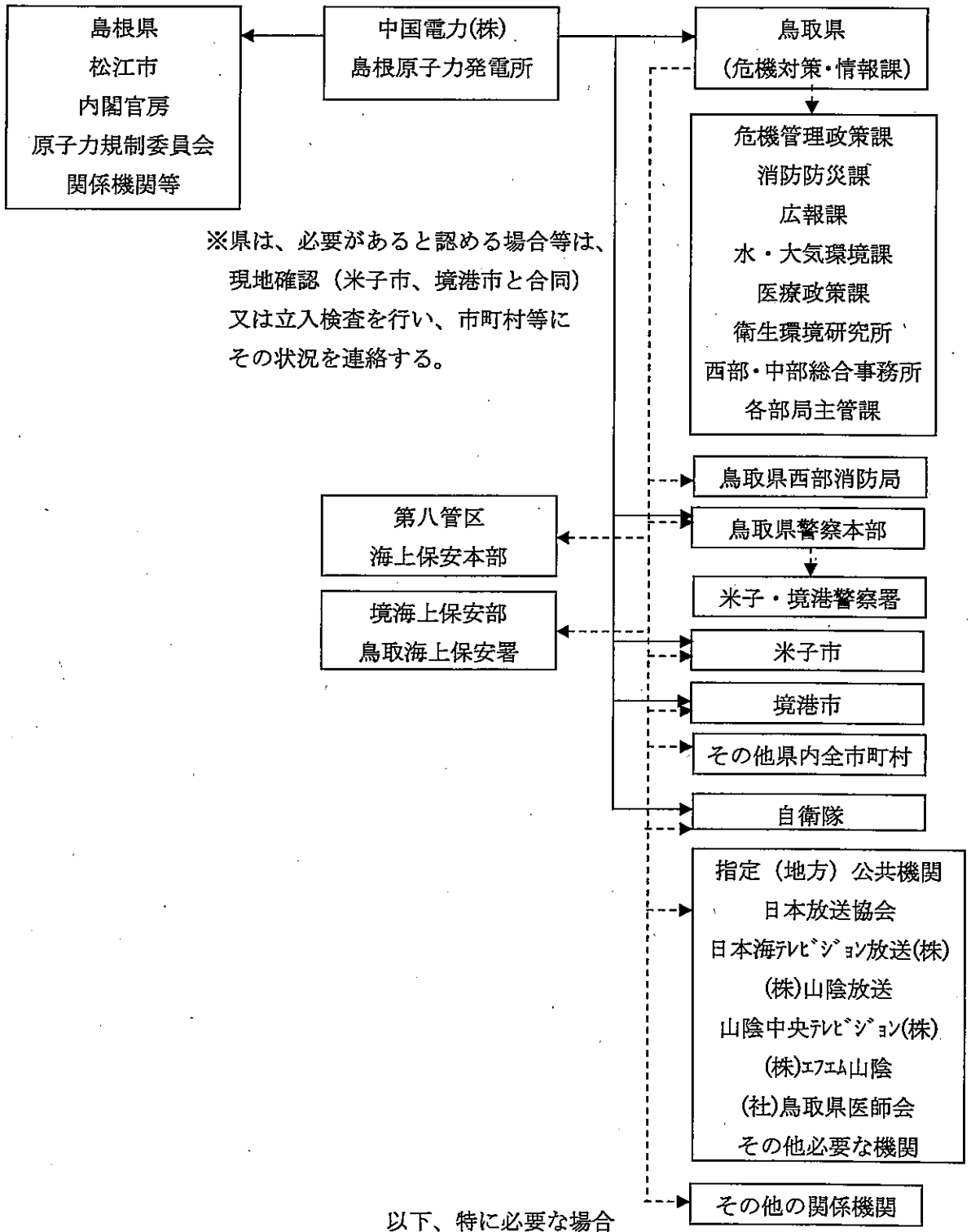
図3-1 特定事象の基準に達しない異常情報等の連絡系統図（島根原子力発電所）
