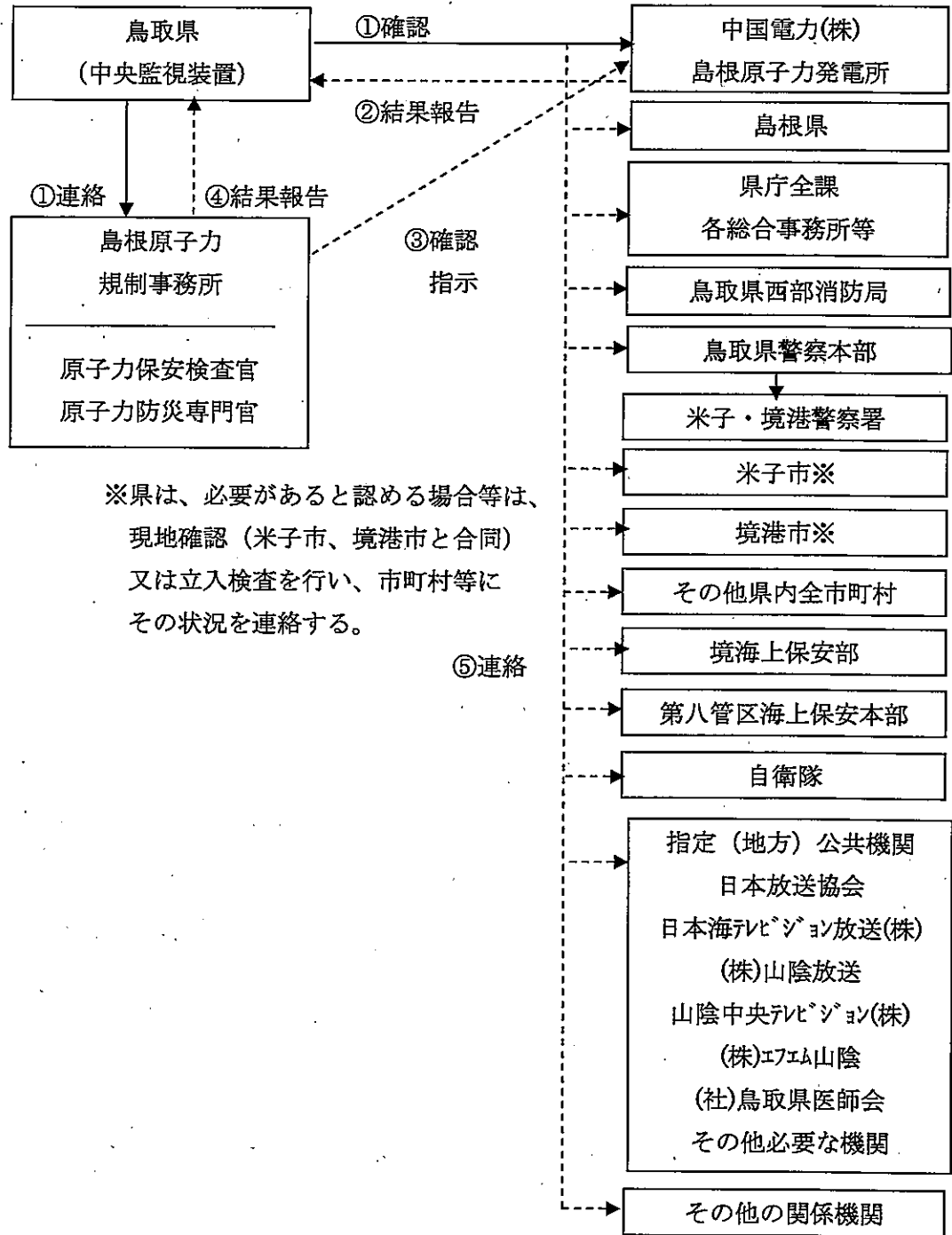
図3-5 県のモニタリングポストで特定事象発生の通報を行うべき数値を発見した場合の連絡系統図（島根原子力発電所）【P：監視装置⇒今年度整備予定】
