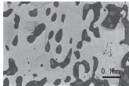
写真49 鉄塊系遺物 (No.26) の外観写真、マクロ、ミクロ組織
