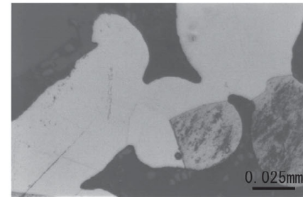
写真47 鉄塊系遺物 (No.11) の外観写真、マクロ、ミクロ組織
