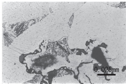
写真48 鉄塊系遺物 (No.16) の外観写真、マクロ、ミクロ組織
