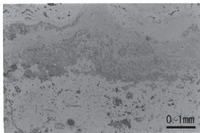
写真43 鉄製品 (No. 8) の外観写真、ミクロ組織
