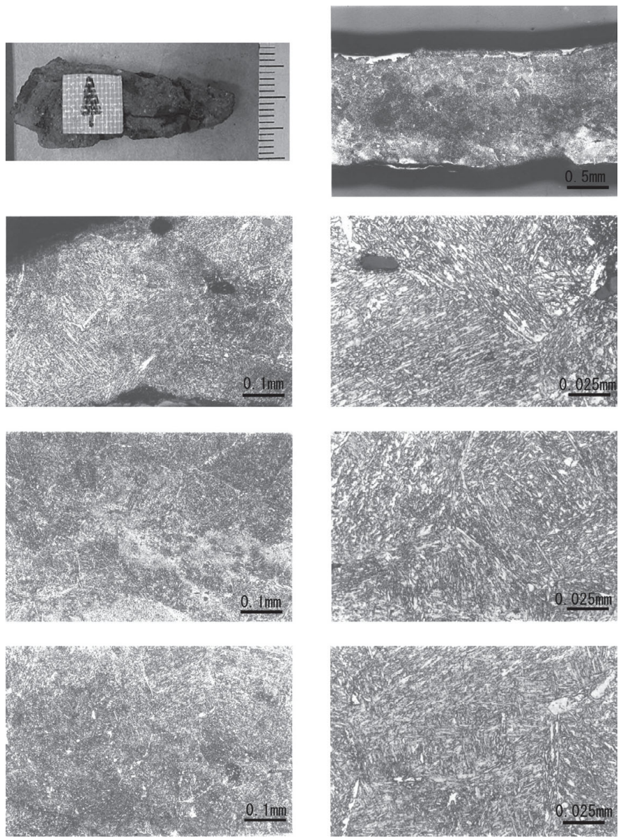
写真45 鉄製品 (No.30) の外観写真、マクロ、ミクロ組織
