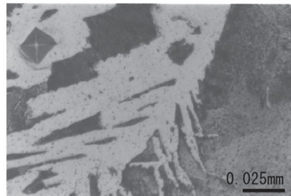
写真46 鉄塊系遺物 (No.9) の外観写真、マクロ、ミクロ組織
