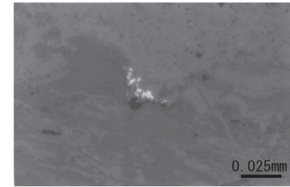
写真44 鉄製品 (No.12) の外観写真、ミクロ組織
