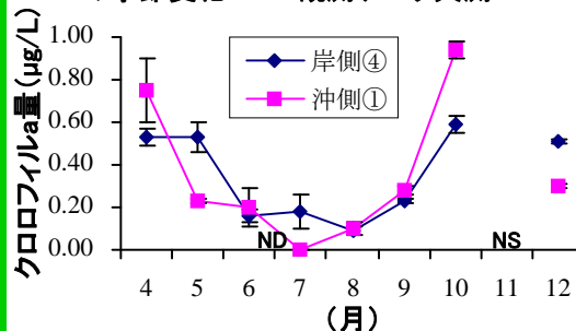
図3) 4～12月の20m以浅のクロロフィルaの平均値の変化. ND: 検出限界以下.
