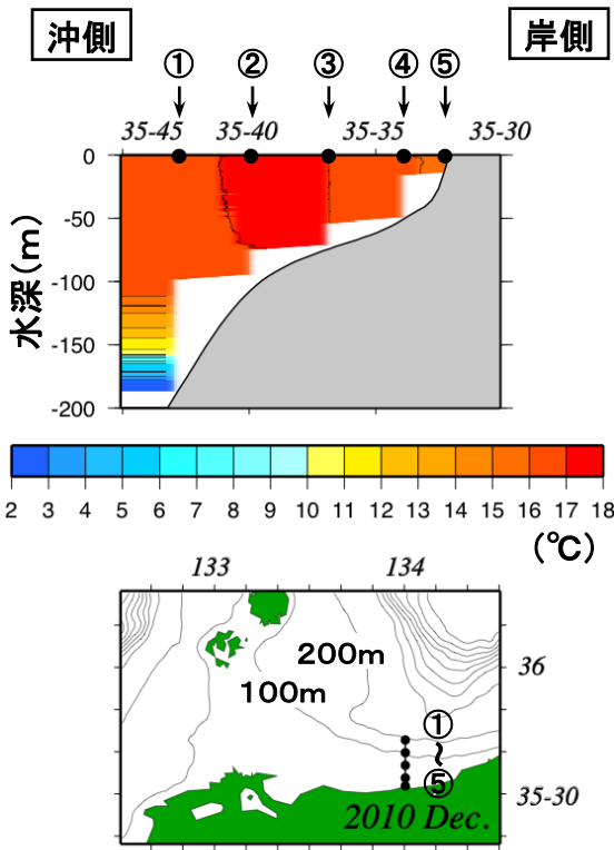
図1) 12月13日の長尾鼻沖における水温の鉛直断面図
