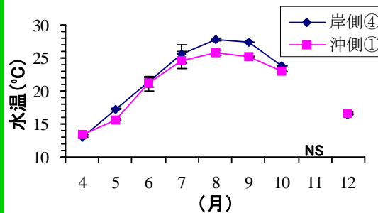
図2) 4～12月の20m以浅の水温の平均値の季節変化. NS: 観測データ欠測.
