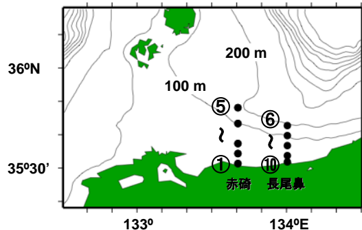
図1) H24年9月5日の調査地点(左)と赤碕(中央)と長尾鼻(右)地先における水温の鉛直分布
