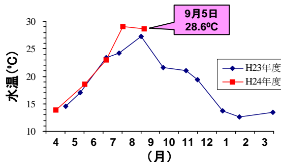
図2) 長尾鼻地先の水深50 m地点(⑨)における海面水温の季節変化。
