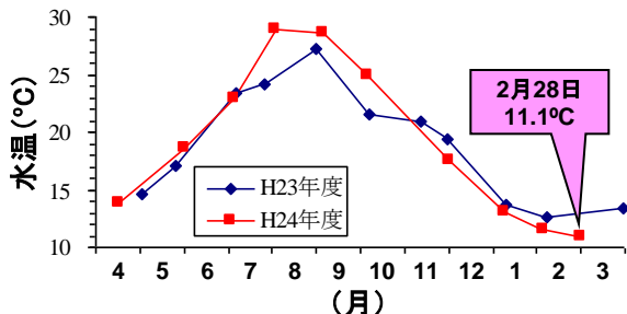
図2) 長尾鼻地先の水深50 m地点(⑨)における海面水温の月変化。
